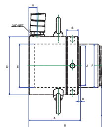
Optional Tilt Saddle (TSA)
